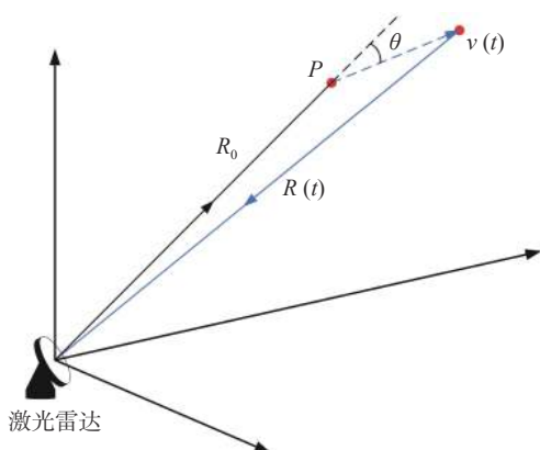
图 1 激光雷达探测原理图
