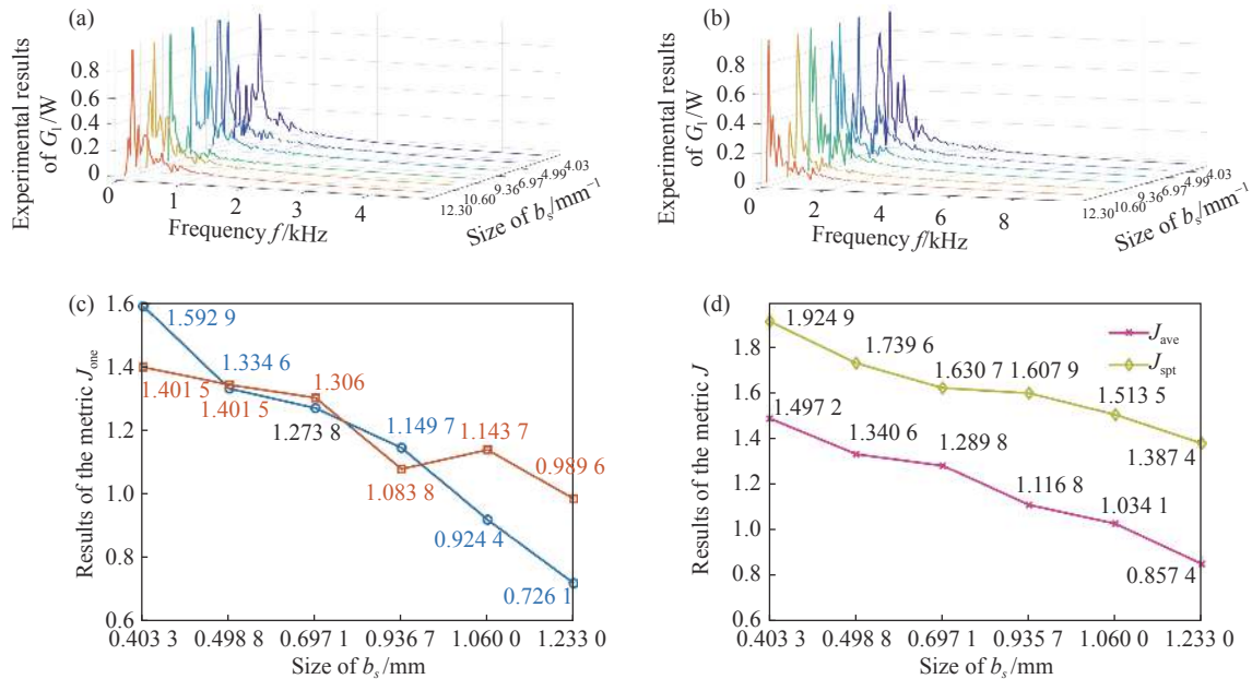
图 8 散斑强度频谱法实验结果, (a)和(b)中横坐标表示强度波动的频率,纵坐标为两个探测器获得的归一化时间频谱。(c)两个单点探测器获得的评价因子 J_{ome} 实验结果, (d)对应两通道的实验结果取平均获得评价因子 J_{ave} 和融合空间时间频谱的评价因子 J_{spt} 。
