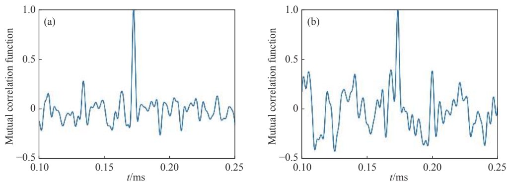
图 3 动态散斑强度波动归一化互相关函数仿真结果。(a) \rho=3 \text{ m} ; (b) \rho=6 \text{ m}
