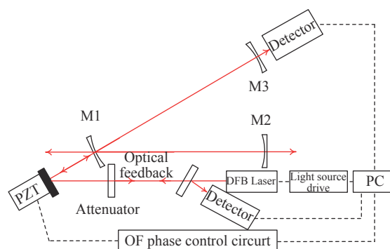
图 10 光反馈腔增强吸收光谱技术原理图
