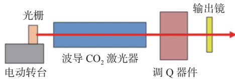
图 1 高峰值功率 CO 2 激光器
