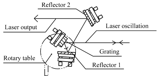
图4 激光器波长调谐系统
