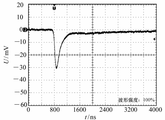
图8 调Q输出激光脉冲波形
