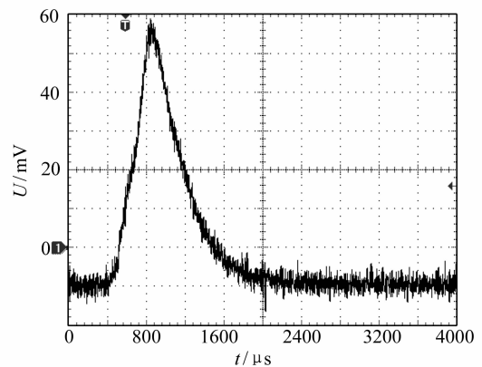
图9 脉冲放电激光脉冲波形
