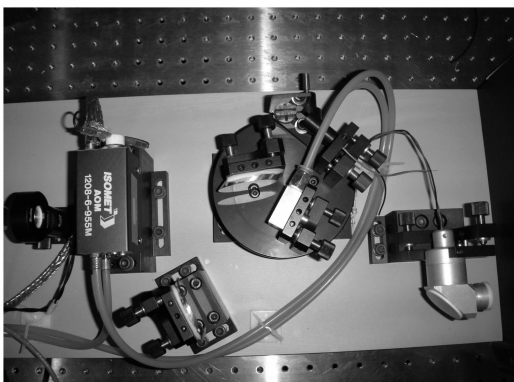
图6 激光器波长调谐系统实物照
