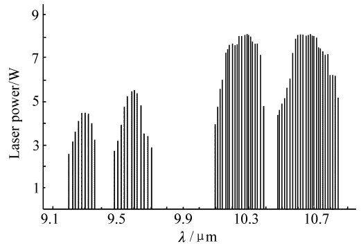
图7 激光输出谱线
