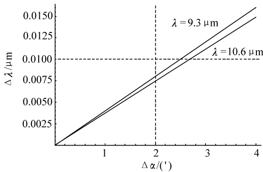
图5 Δλ 与 Δα 的关系
