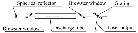
图 2 一级振荡、零级输出 CO 2 激光器谐振腔 Fig. 2 First-order oscillating and zero-order output CO 2 laser cavity
