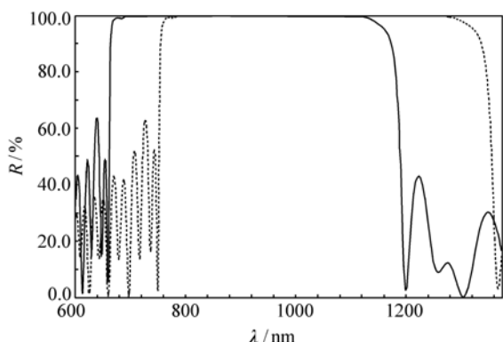
图3 高反射膜的光谱理论反射率曲线
