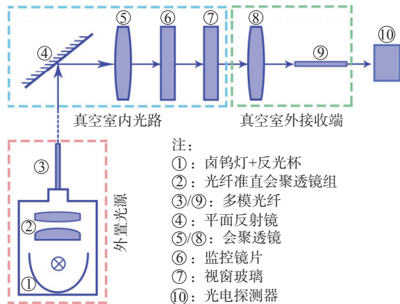
图 4 光路系统原理 Fig. 4 Schematic of the Optical Path System
