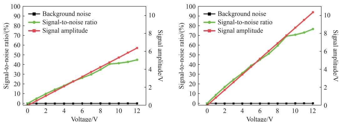
图 12 底噪、信噪比与信号幅值关系曲线
