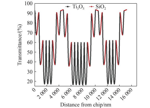
图 17 膜层监控曲线 Fig. 17 Film layer monitoring curve
