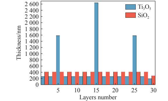
图 16 膜厚结构柱状图 Fig. 16 Bar chart of film thickness structure
