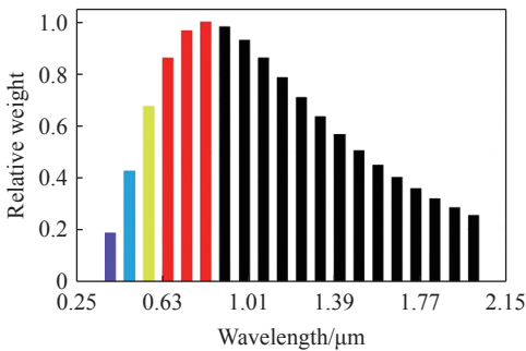
图 5 光源光谱图 Fig. 5 Light source spectrum
