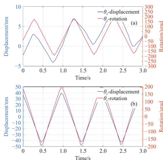
图14 转动-平动耦合系数标定。(a)绕 x 轴转动的转动角度 \theta 和耦合误差 \delta L ; (b)绕 y 轴转动的转动角度 \theta 和耦合误差 \delta L
