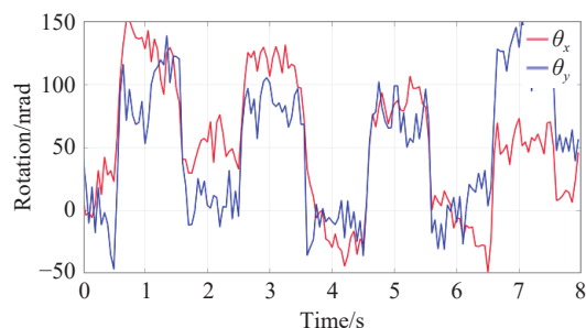
图 10 干涉光路绕 x 轴和绕 y 轴转动的分辨率
