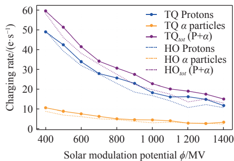
图2 检验质量在轨充电速率
