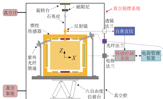
图 10 电荷管理地面测试系统示意图
