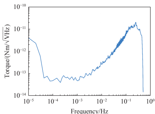
图 12 扭摆的力矩分辨率
